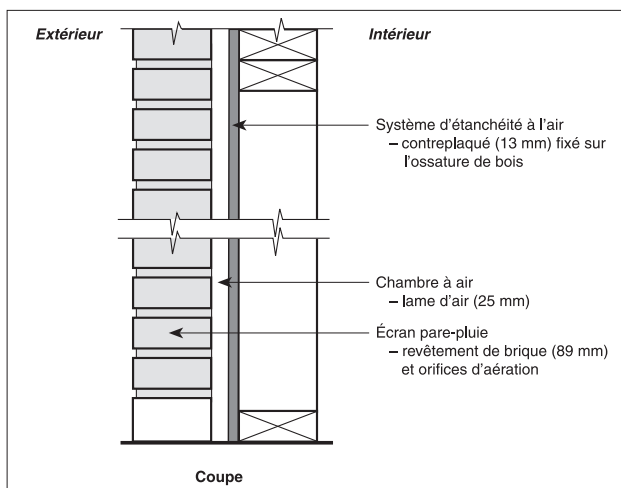
Figure 5. Exemple de mur flexible
