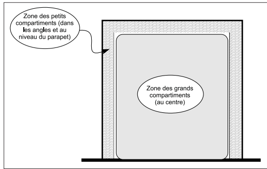
Figure 3. Schéma général de compartimentation des façades
